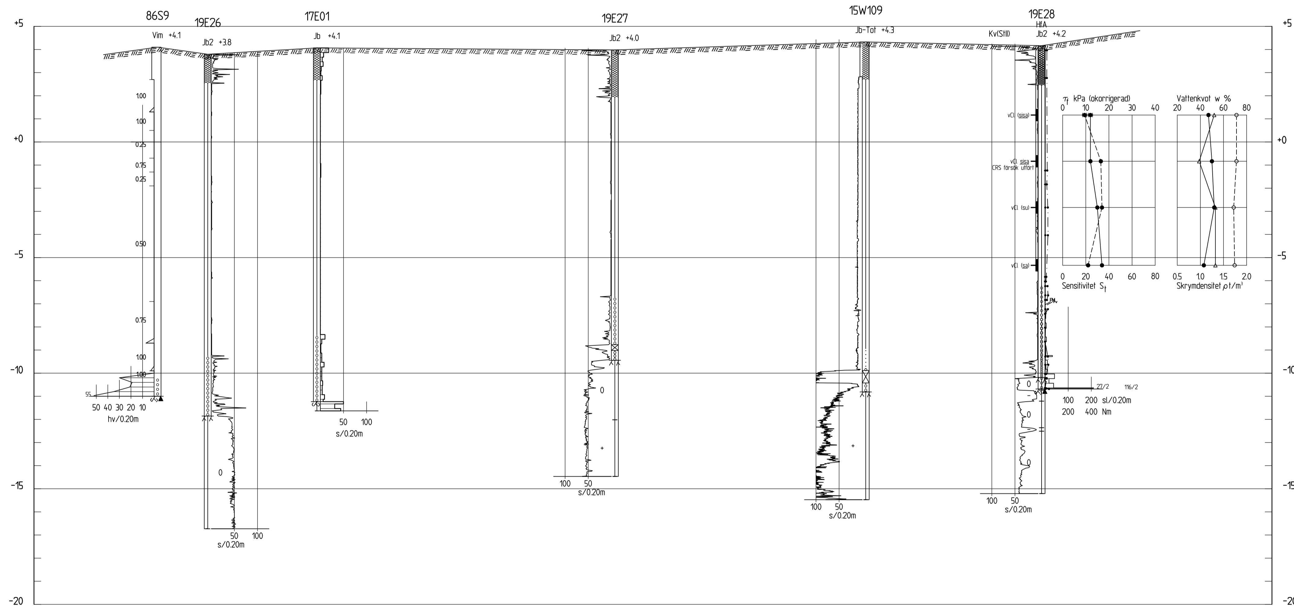
SEKTION C-C 1:100
