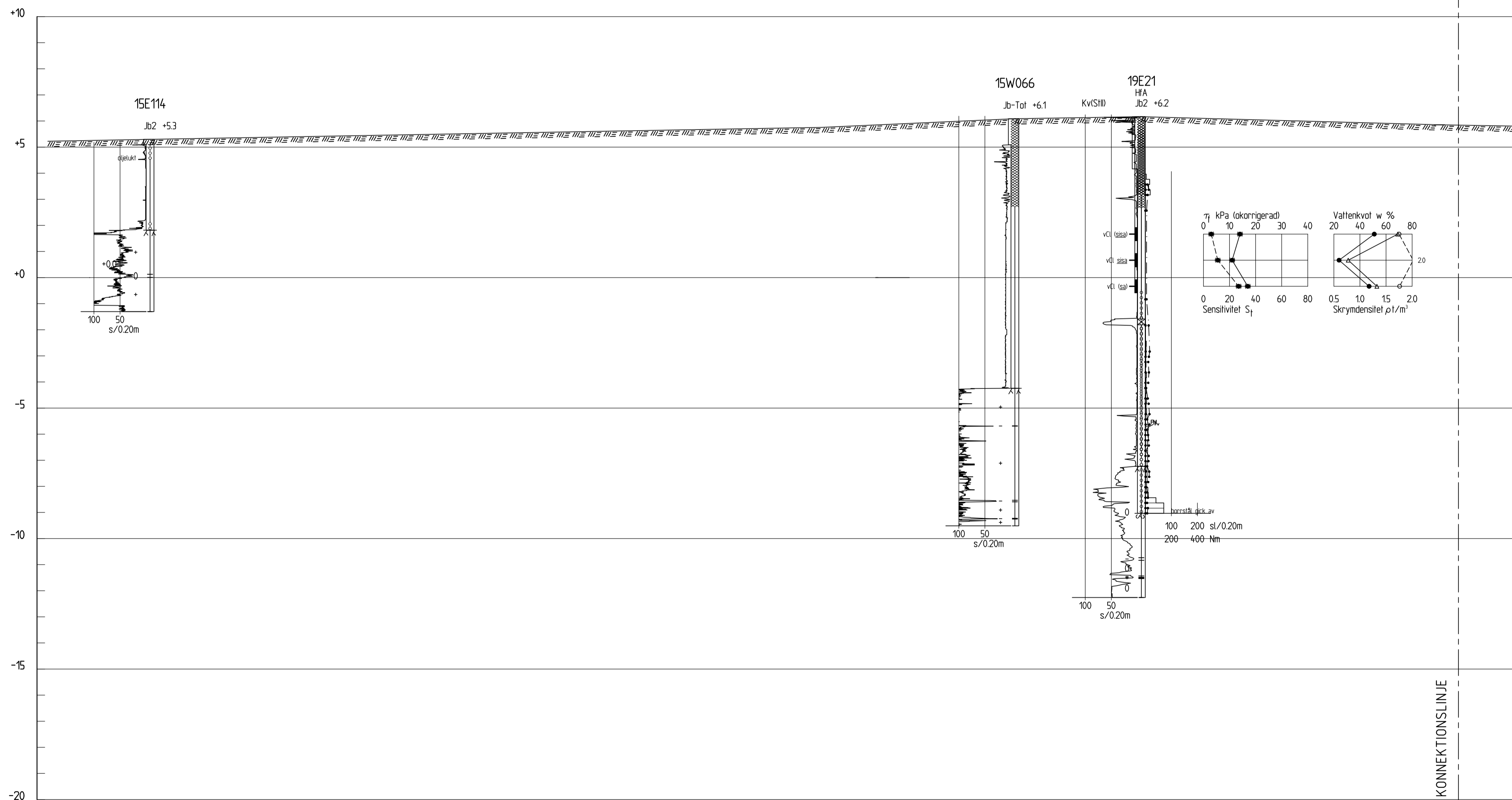
SEKTION B-B 1:100
