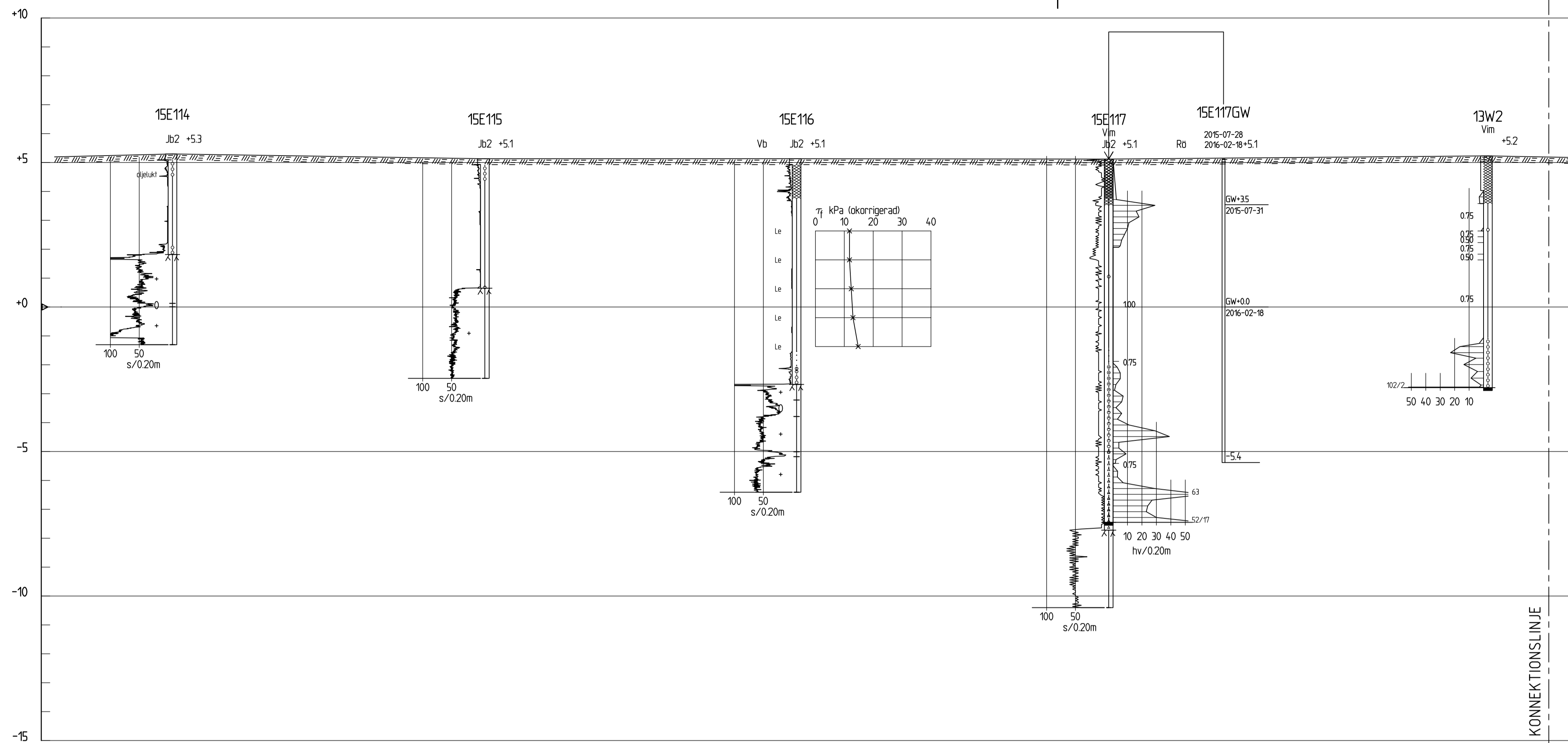
SEKTION A-A 1:100
