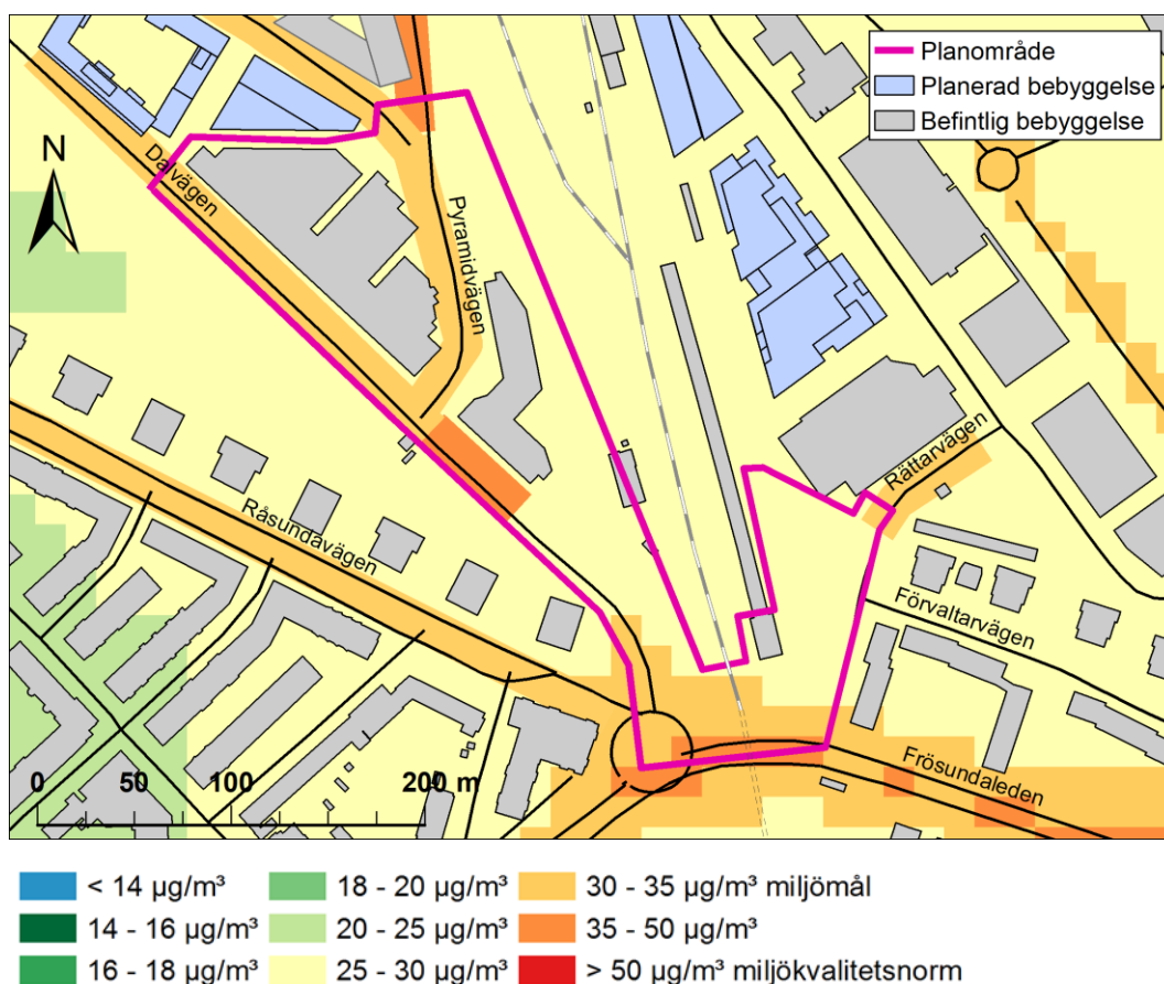
Figur 5. Beräknad dygnsmedelhalt av partiklar, PM10 ( \mu\text{g}/\text{m}^3 ) under det 36:e värsta dygnet för nollalternativet år 2025. Normvärdet som ska klaras är 50 \mu\text{g}/\text{m}^3 .
